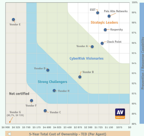
Figure 4: EPR CyberRisk Quadrant™ by AV Comparatives
